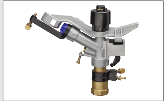
Irrigatore "Jenny" settore bigetto 1" femmina Irrigator "Jenny" 1" female sector - 2 jet
