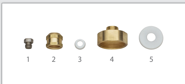
Esploso ghiera completa per lance modello economico Economical spray gun nut exploded
